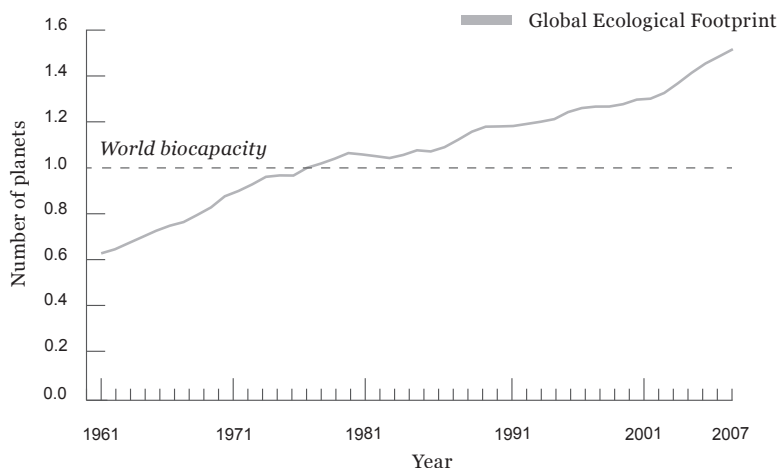
Figuur 4: Gebruik van de biocapaciteit Bron: Living Planet Report 2010 , Geneva, 2010, WWF
