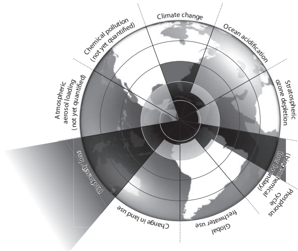
Figuur 6: Rockström: planetaire grenzen
