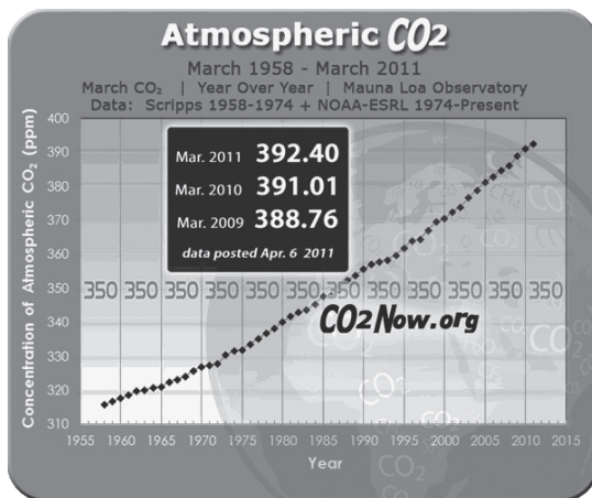
Figuur 5: \text{CO}_2 stijging Bron: co2now.org
