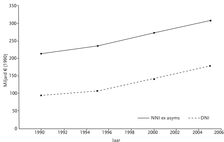
Figuur 2: DNI Nederland en het NNI Nederland, 1990-2005
